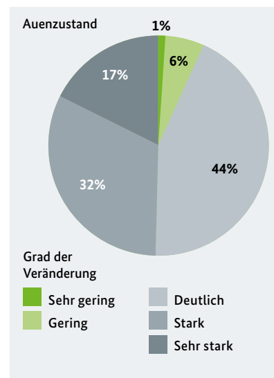
Abb. 3: Verteilung der Zustandsklassen rezipienter Auen an Bundeswasserstraßen
